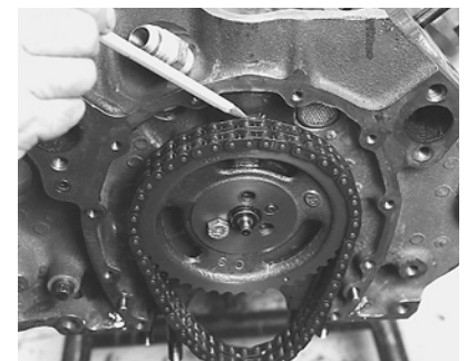
Figura 2 - Revise el alineamiento de la cadena para asegurarse que ambas ruedas dentadas estén correctamente instaladas
